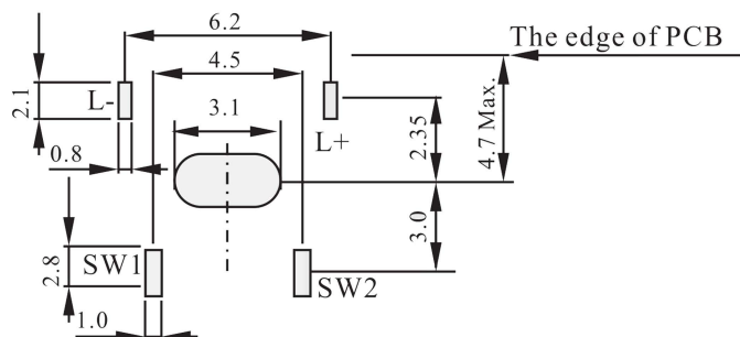
SMD type - SPJT
