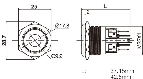
RJS103-22L(A)-F-D~67J
