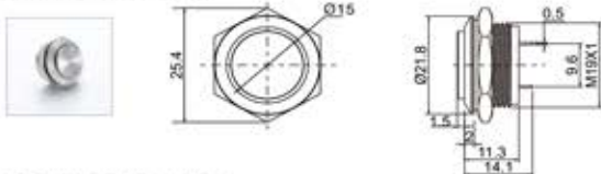
RJS1N1LP-25M-H~67J
