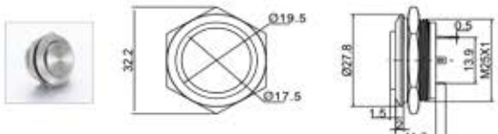
RJS1N1LP-25M-H~67J
